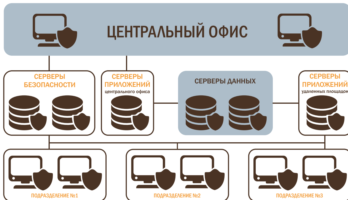
Схема «Корпоративная информационная система»
